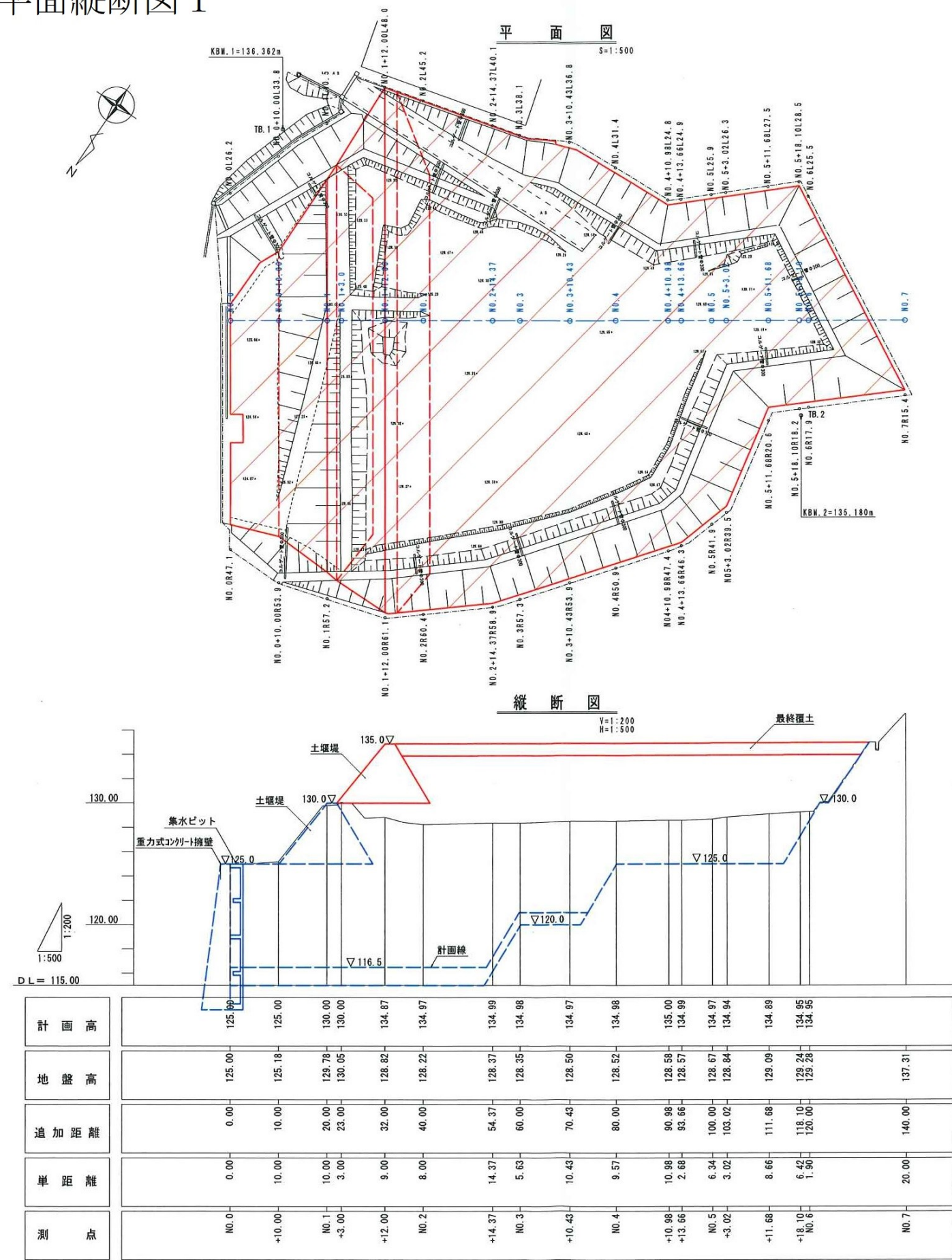
平面縦断図 1
